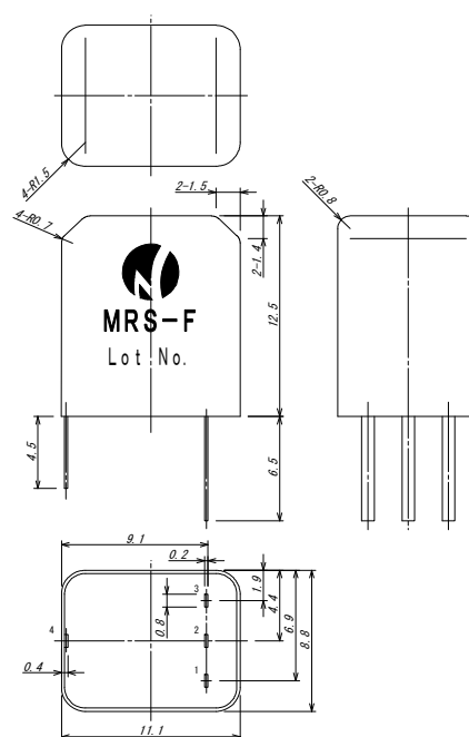
外形図
